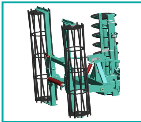
Hidraulički stražnji nosač u 3 točke za kultivatore i valjke, itd. Hydraulic rear carrier a three point for cultivators and rollers, etc. Porte-outils arrière à 3 points hydraulique pour les rouleaux ou cultivateurs Portaherramientas trasero hidráulico de tres punto para rodillos y coltivadores.
